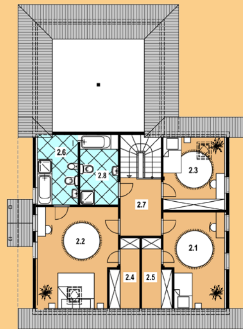
PODDASZE
