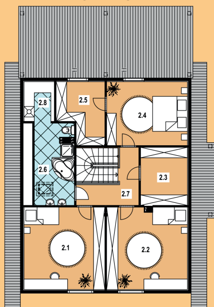
PODDASZE
